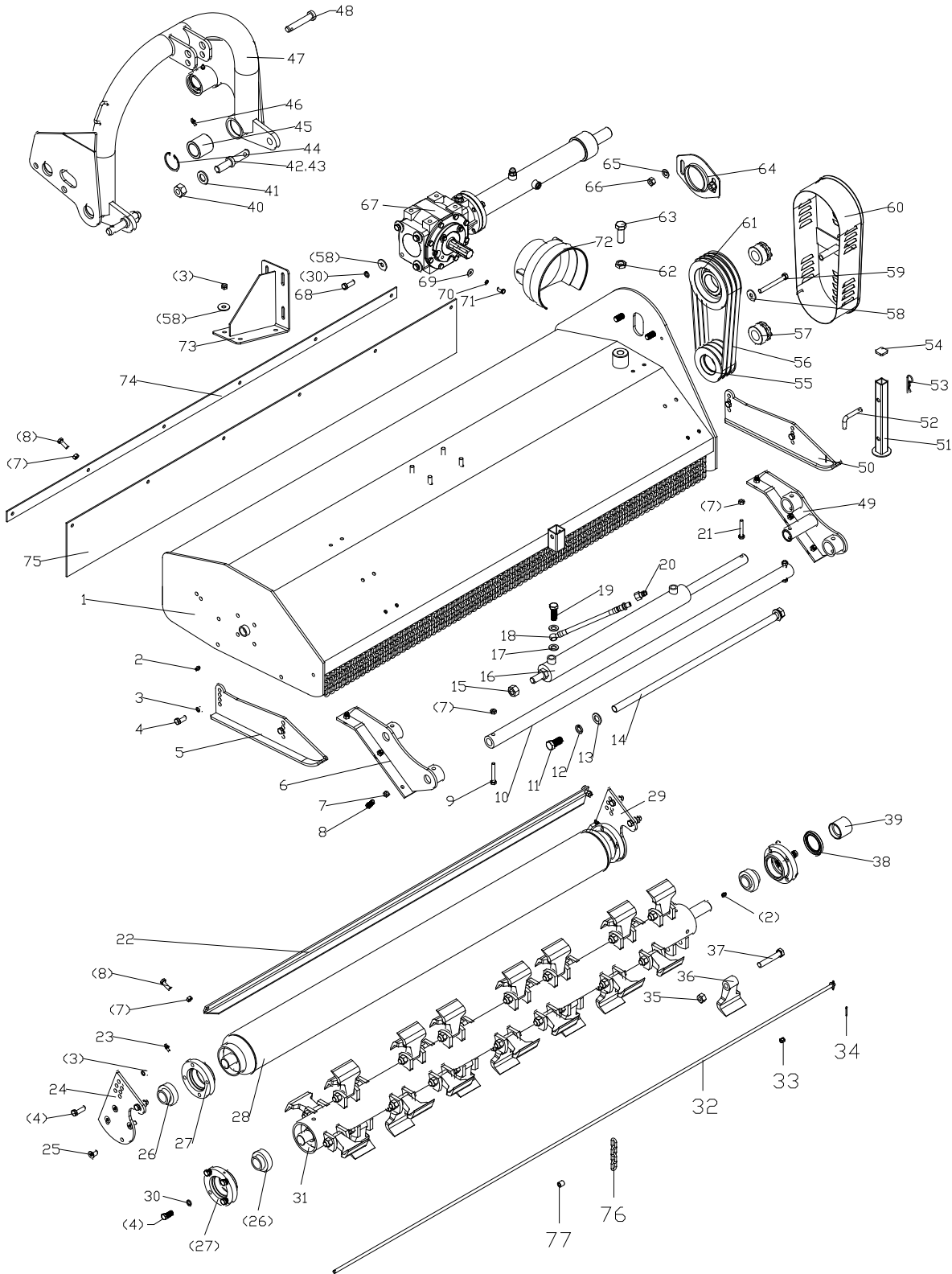
Fig. 1 Huvudmaskin
