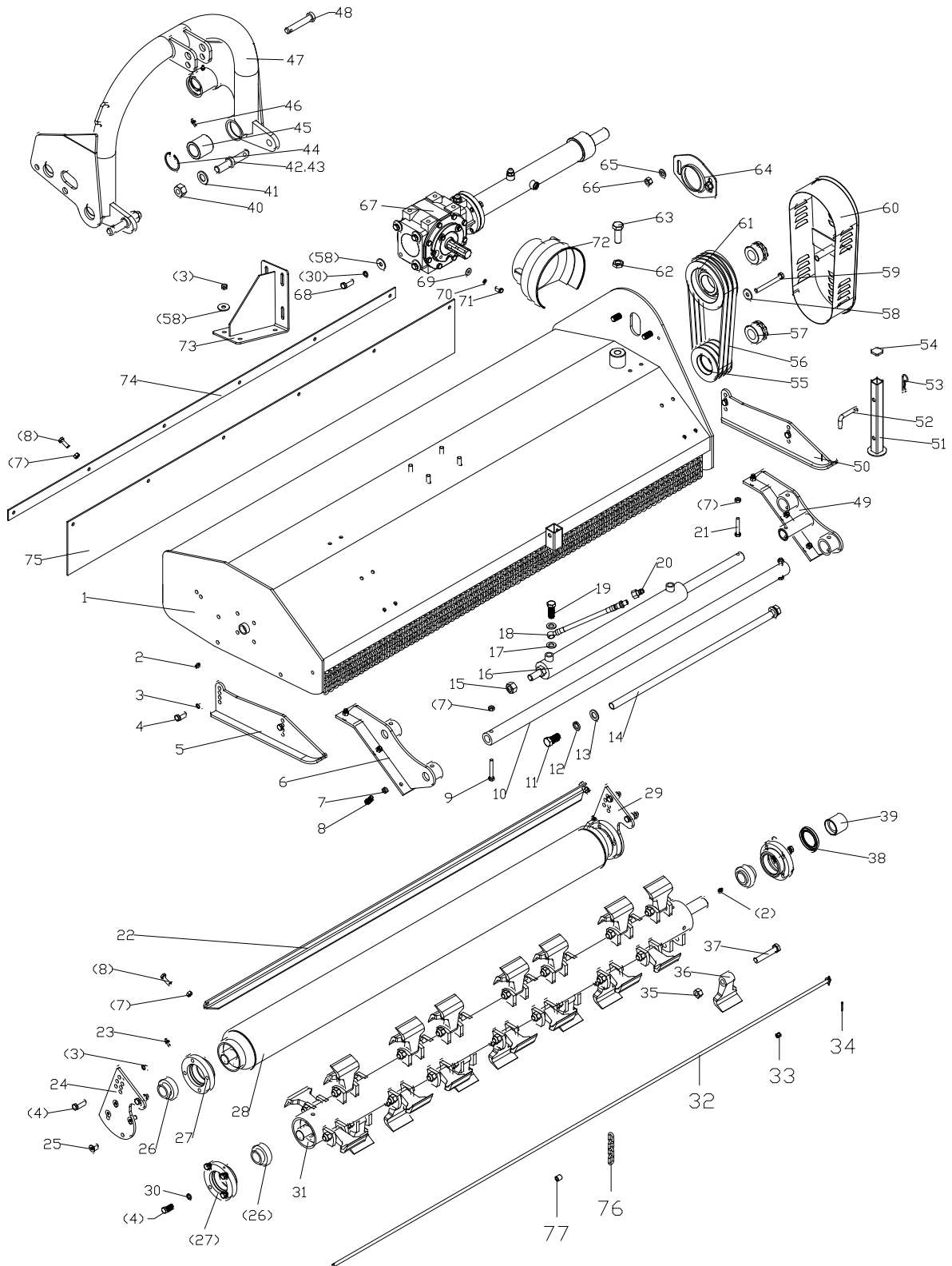
Abb. 1 Hauptgerät
