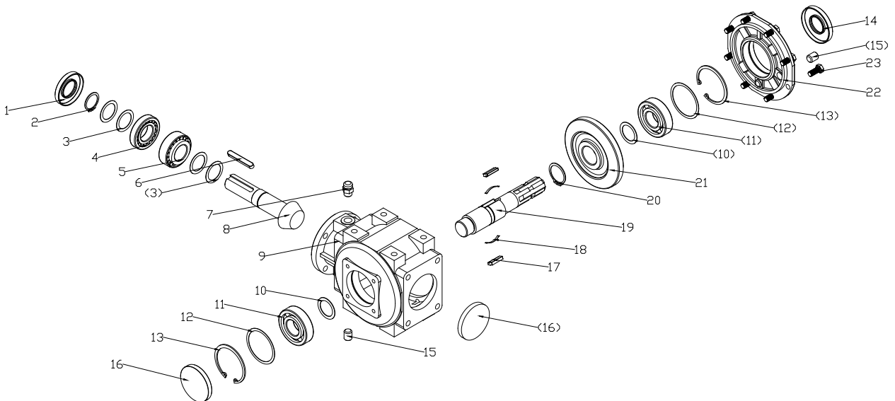
Fig. 3 - Gearkassedele
