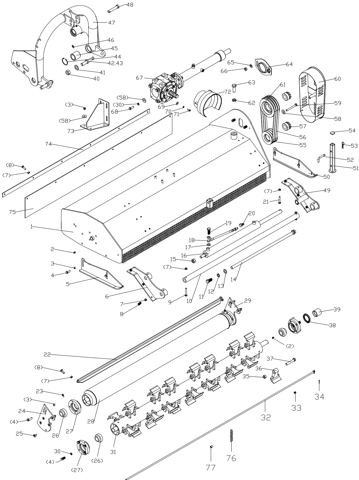
Fig. 1 Hovedmaskine
