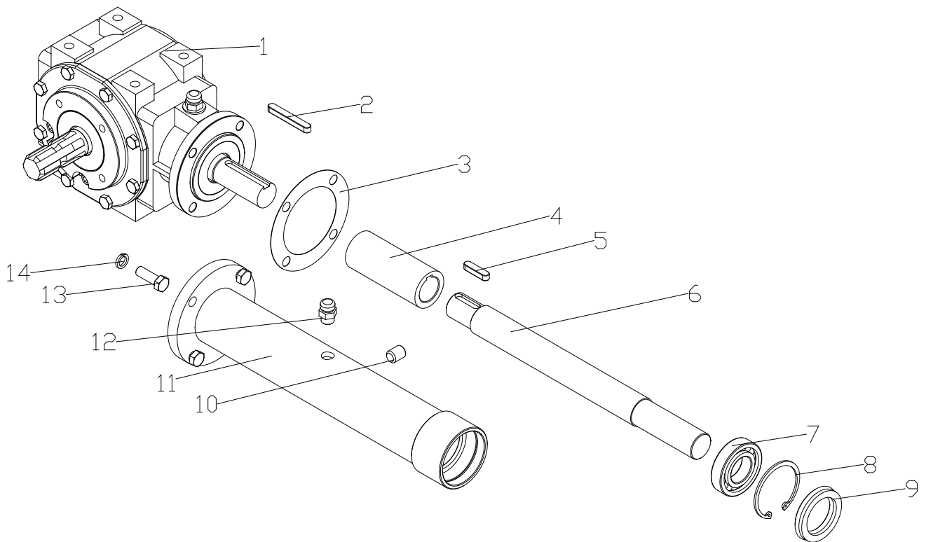
Fig. 3 - Gearkassedele
